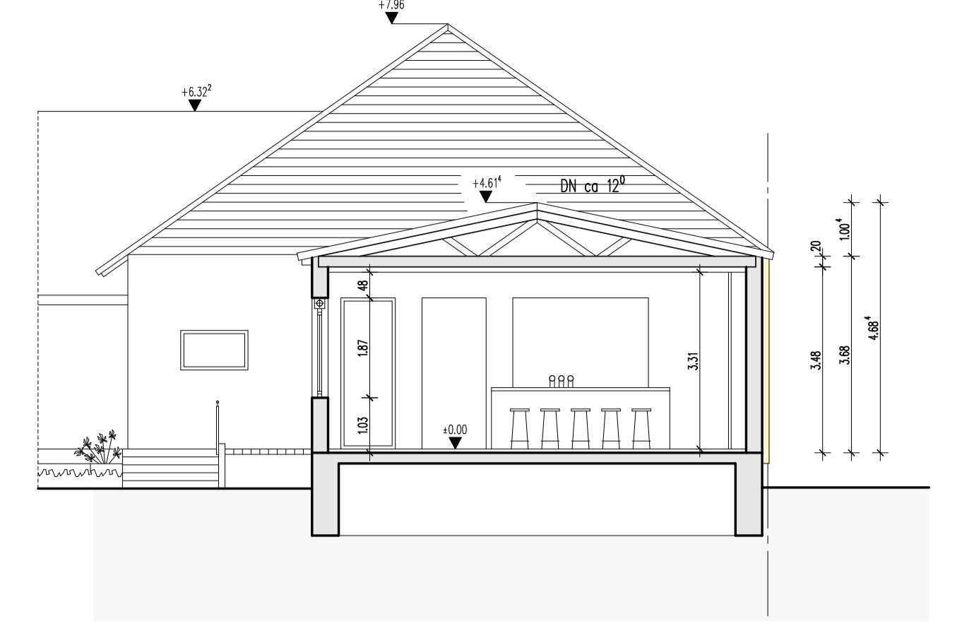
SCHNITT B - B
