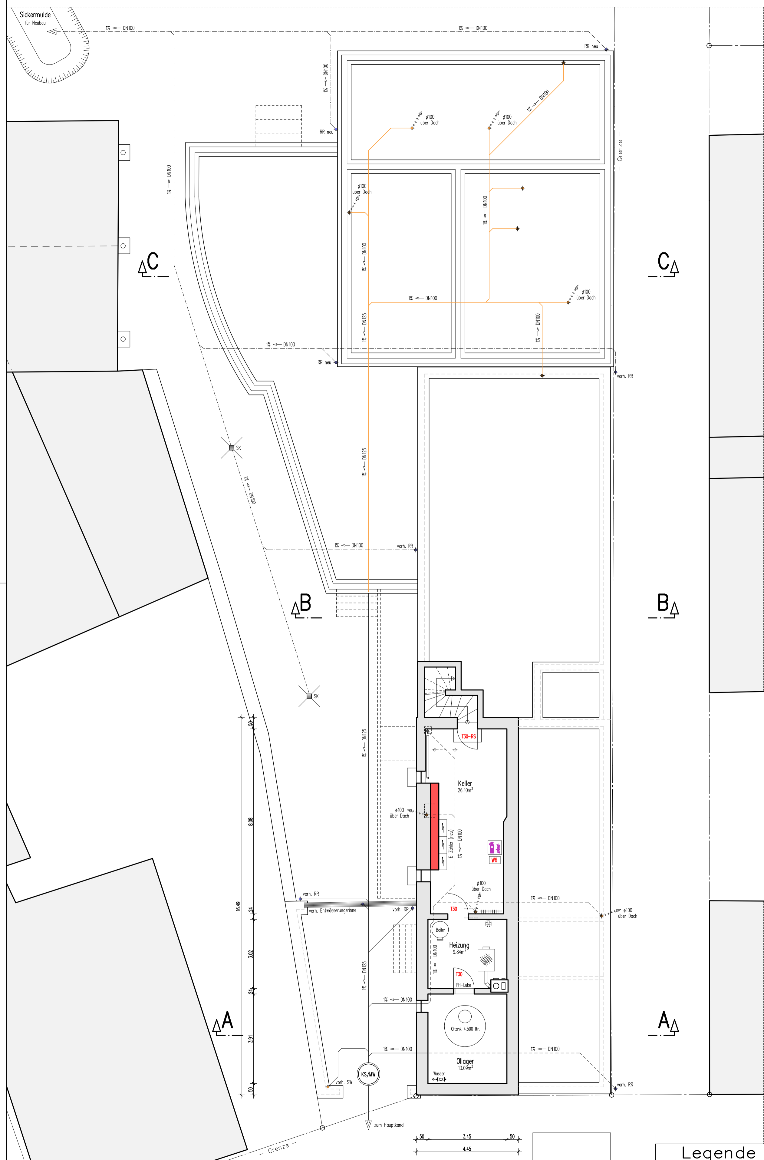
KELLERGESCHOSS
