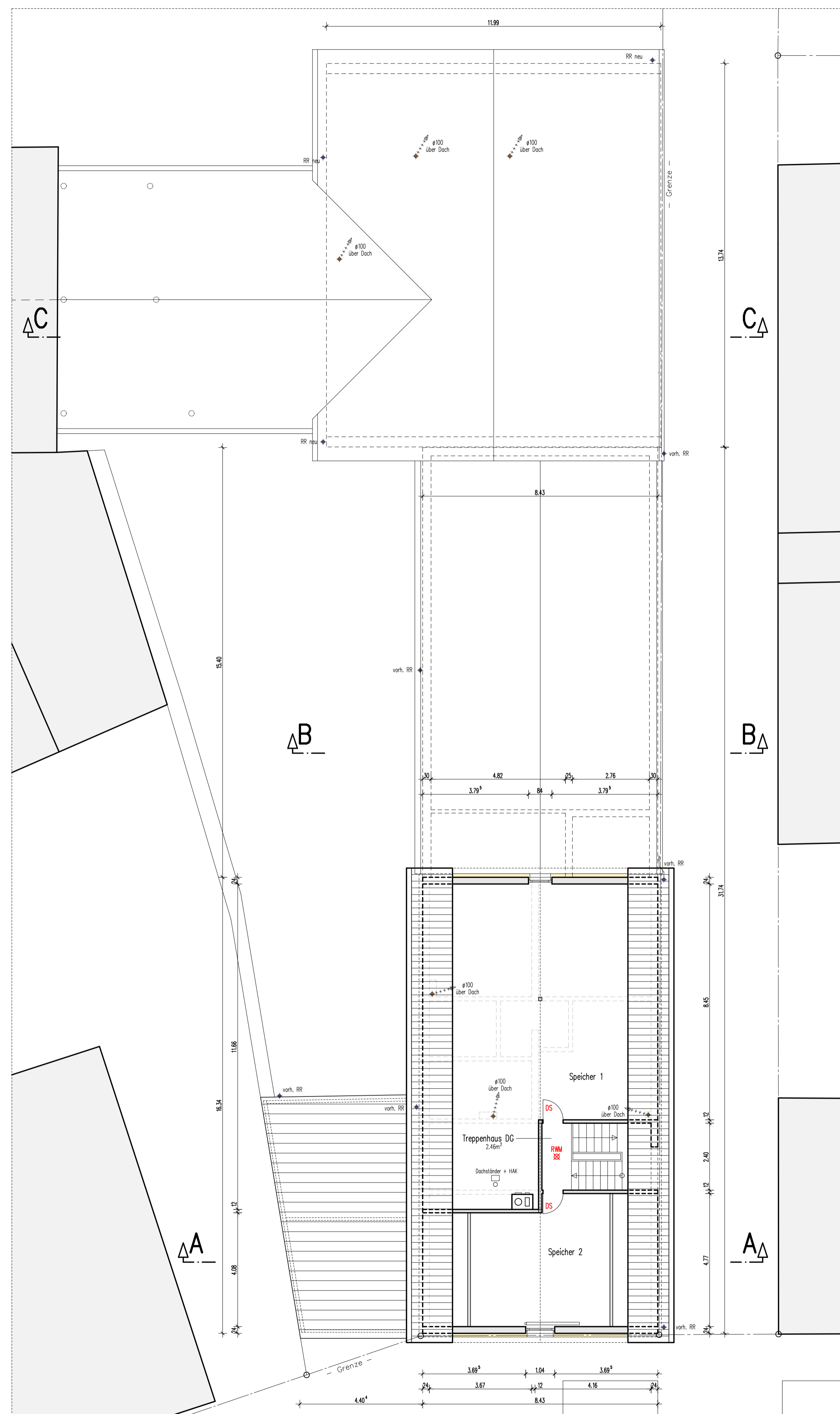
DACHGESCHOSS
