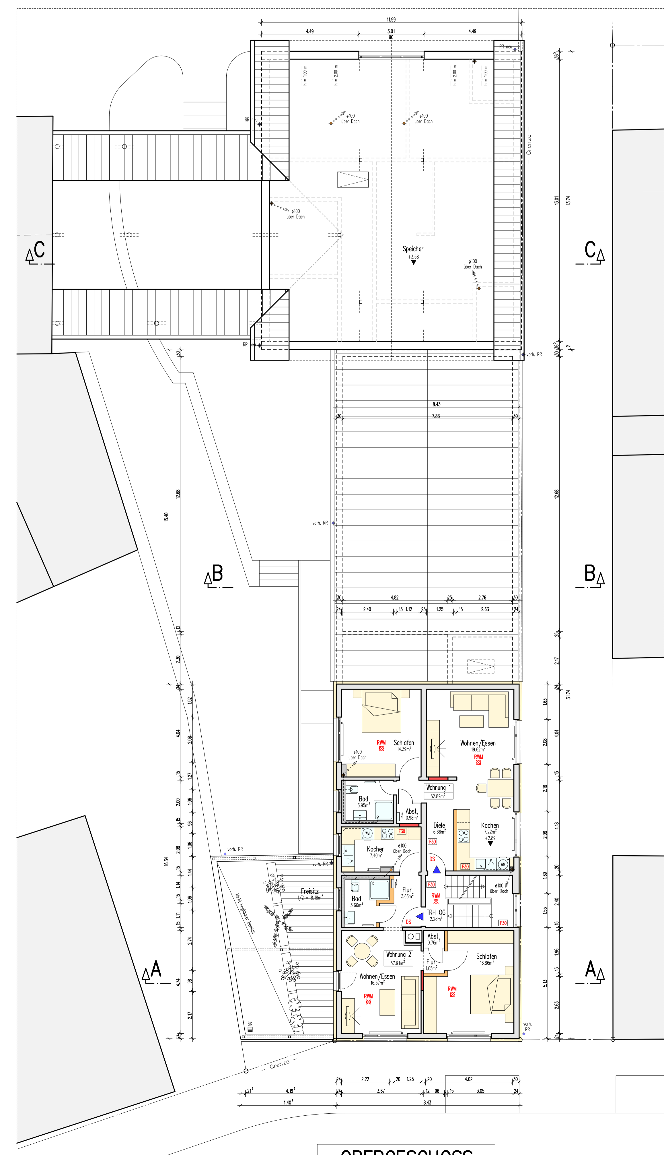
OBERGESCHOSS
